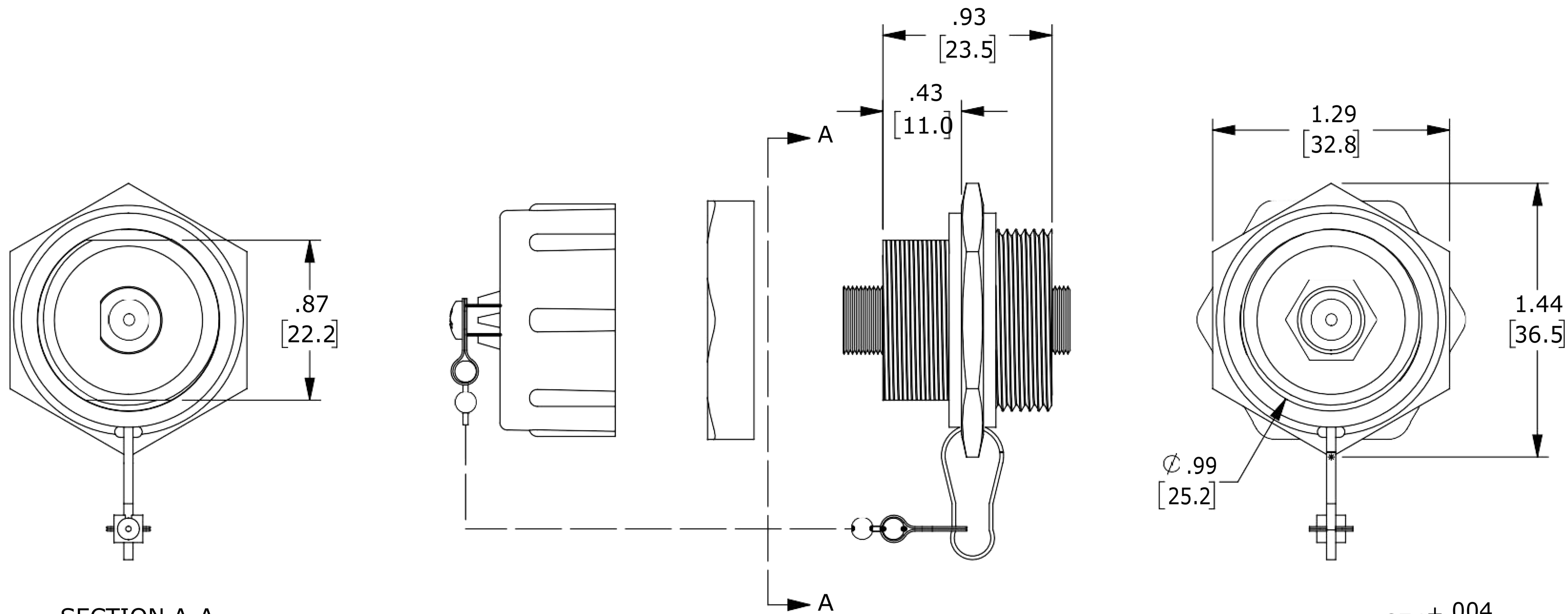
SECTION A-A
